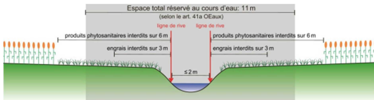
Fig. 2. Exemple de délimitation de l'ERE pour les petits cours d'eau. Quand l'ERE est fixé, la largeur des bandes tampon selon l'ORRChim et l'OPD se mesure depuis la ligne de rive.
