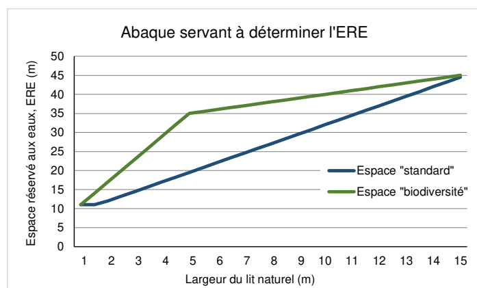
Fig. 1. Abaque pour la détermination de l'ERE.
