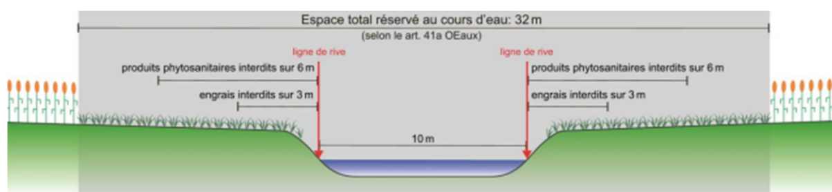
Fig. 3. Exemple de délimitation de l'ERE pour un cours d'eau d'une largeur de 10 m.
